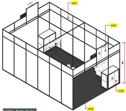
Isométrica - Esquina • Esquina ESCALA 1:25
