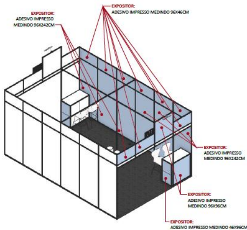
Comunicação Visual - Para Expositor | Esquina • Esquina ESCALA 1:25
