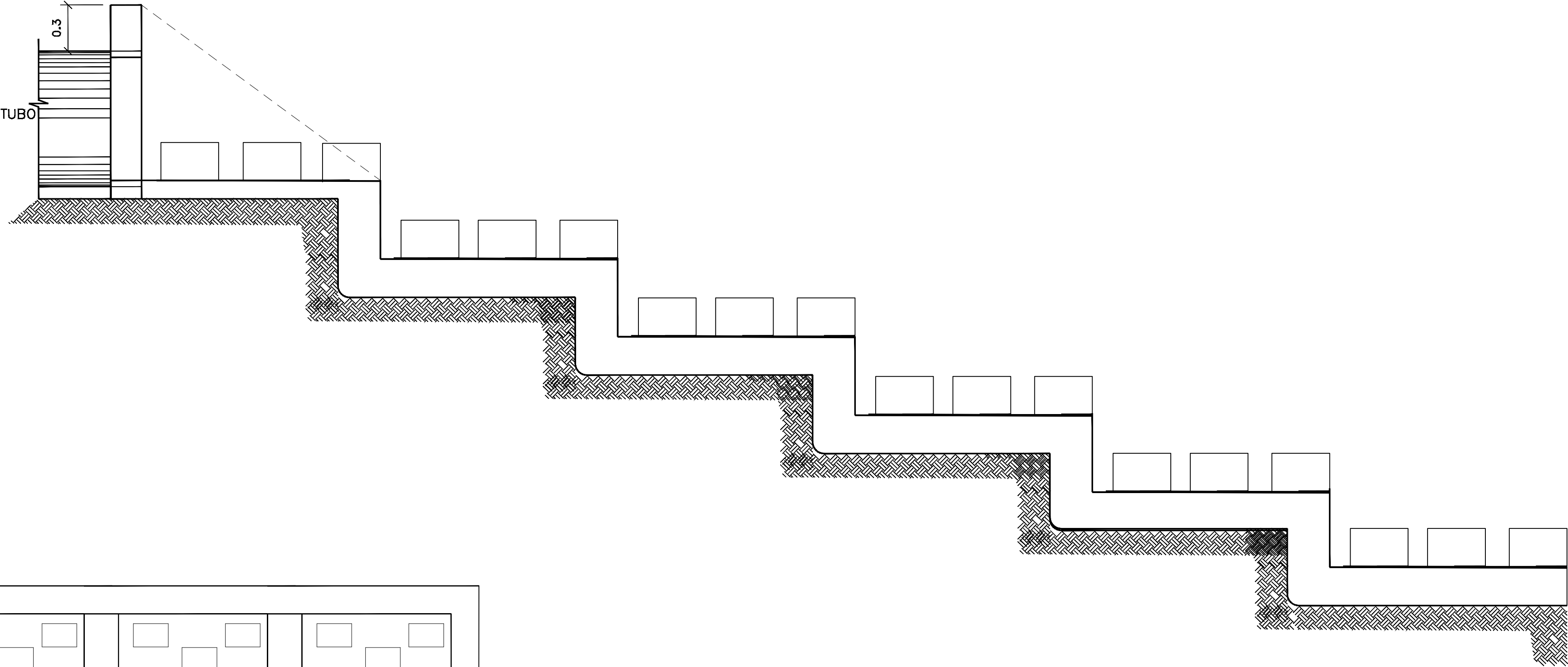
Corte A-A
