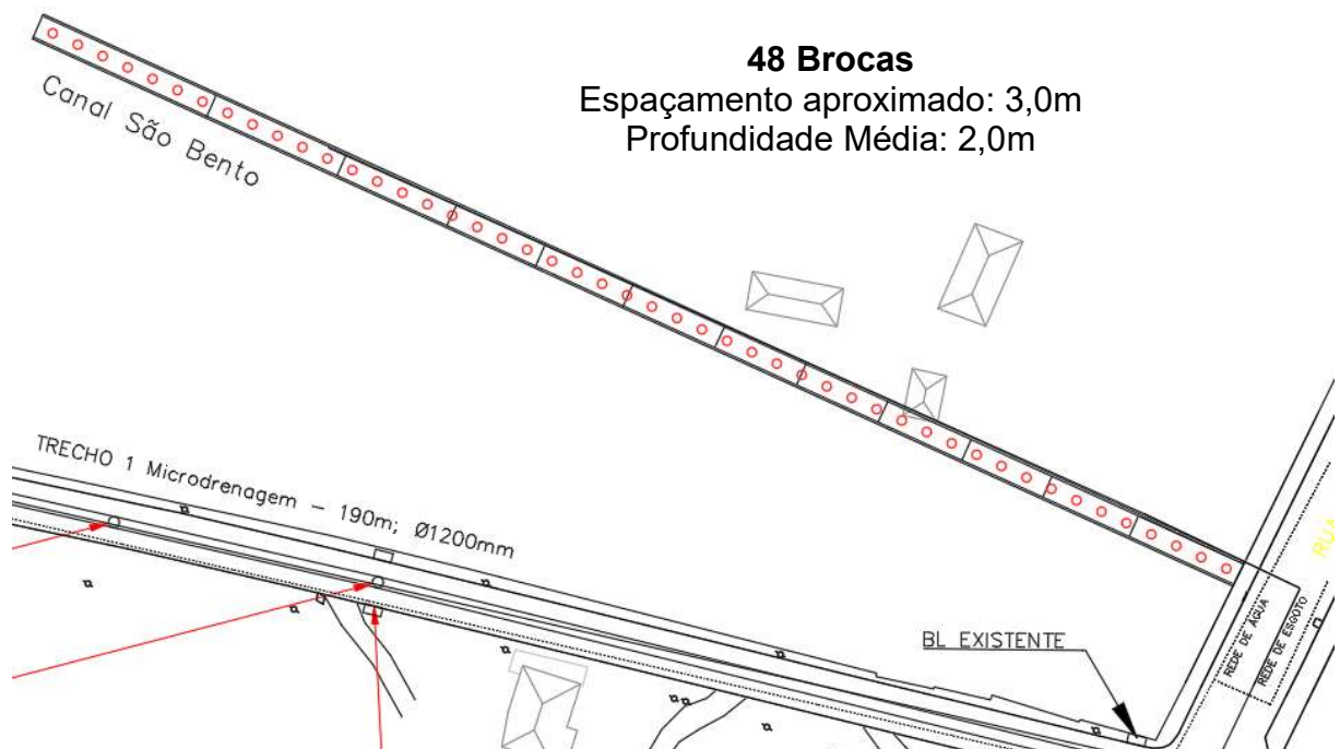
Figura 4 – Quantitativo de brocas de fundação para o canal/escada hidráulica no córrego São Bento
