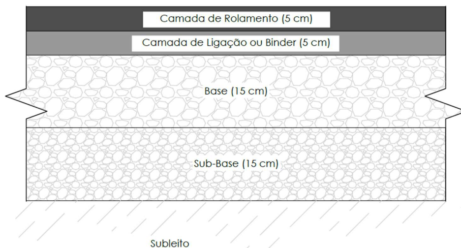
Figura 9 – Seção transversal típica do serviço de recomposição de pavimento
