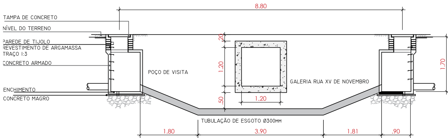
SIFÃO INVERTIDO - PERFIL LONGITUDINAL ESC 1:75
