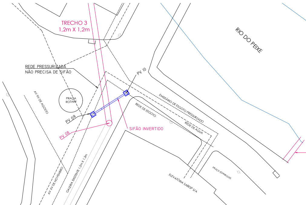
IMPLANTAÇÃO SIFÃO INVERTIDO ESC 1:500
