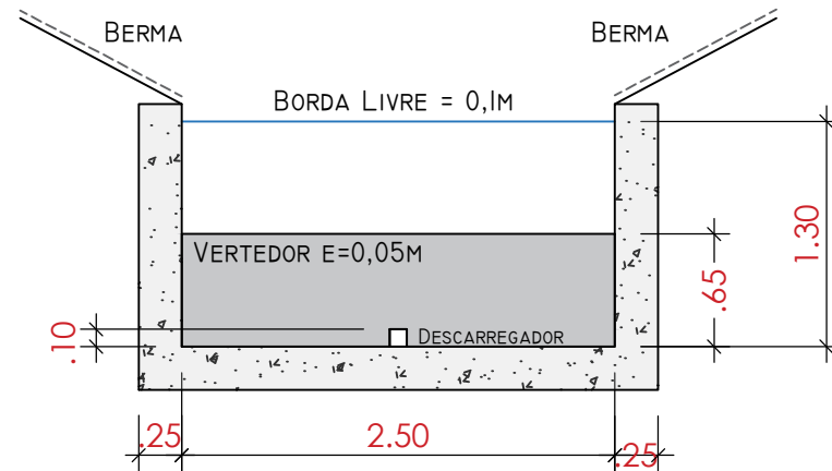
CANAL SÃO BENTO - SEÇÃO TRANSVERSAL ESC 1:50
