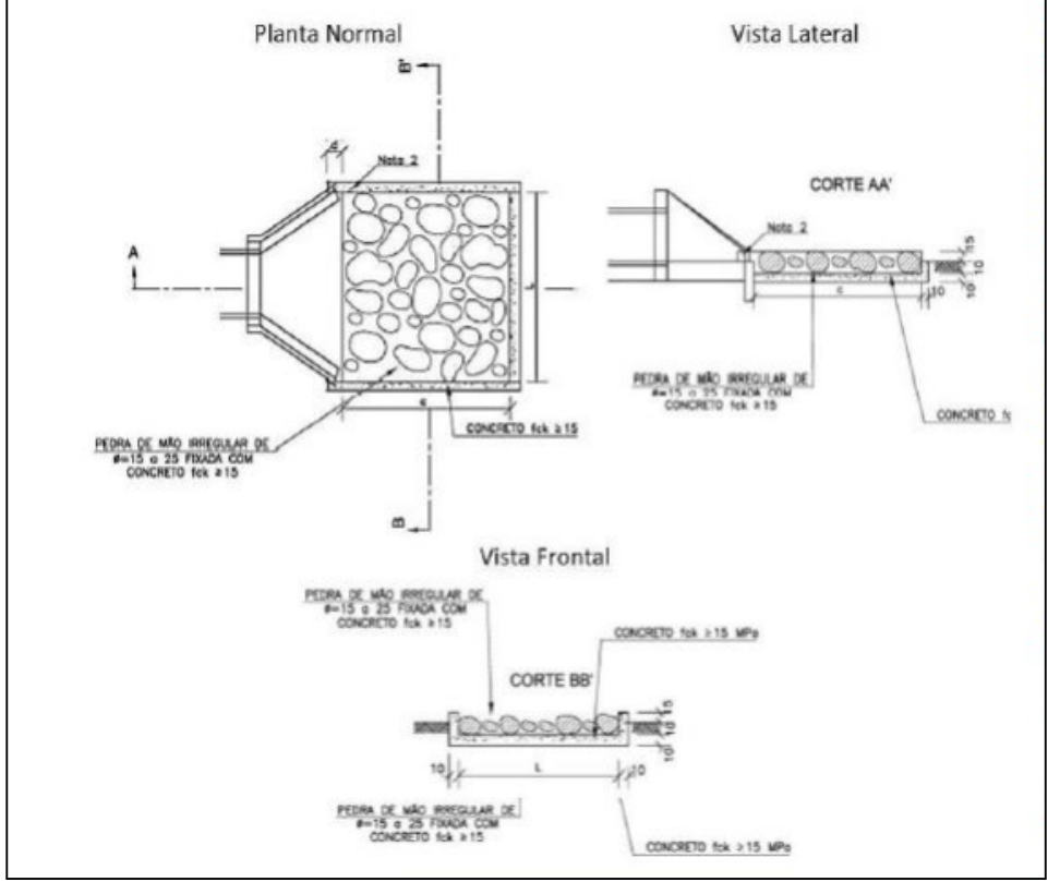
DETALHES - BACIA DE DISSIPAÇÃO SEM ESCALA
