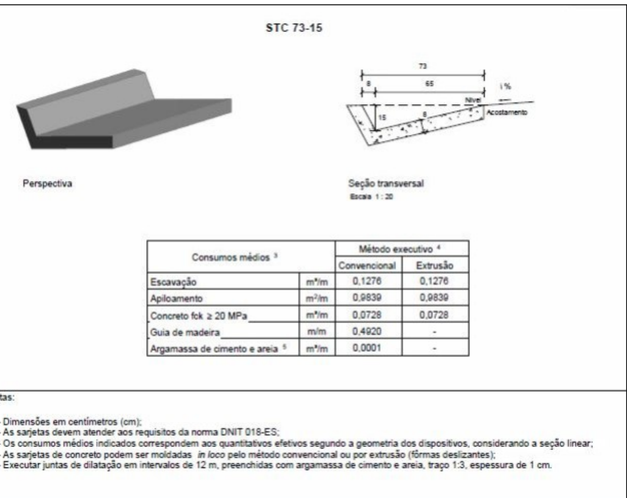
DETALHES - SARJETA TRIANGULAR DE CONCRETO - STC 73-15 SEM ESCALA
