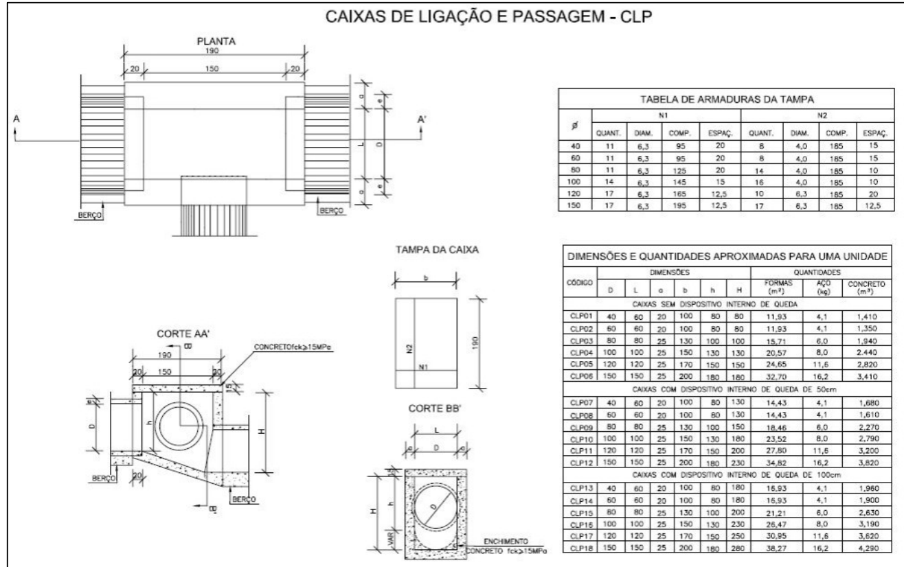
DETALHE - CAIXA DE LIGAÇÃO E PASSAGEM - CLP SEM ESCALA
