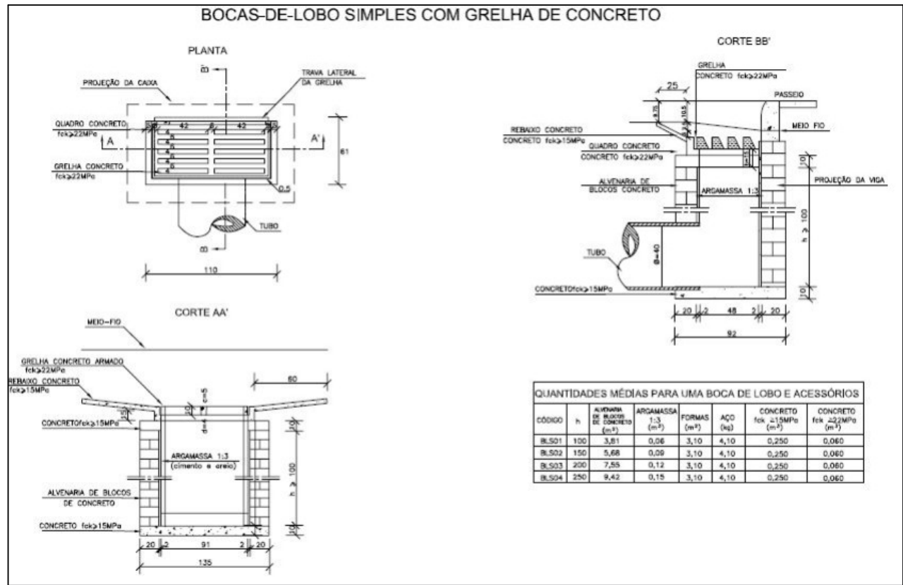
DETALHE - BOCA DE LOBO SIMPLES - BLSG SEM ESCALA
