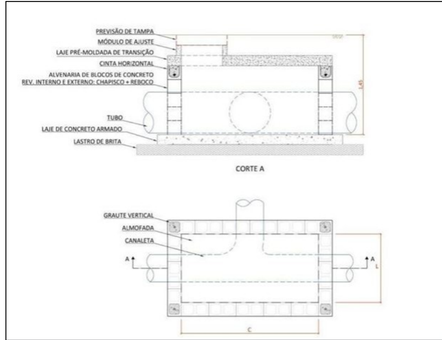
DETALHES - BACIA DE DISSIPAÇÃO SEM ESCALA
