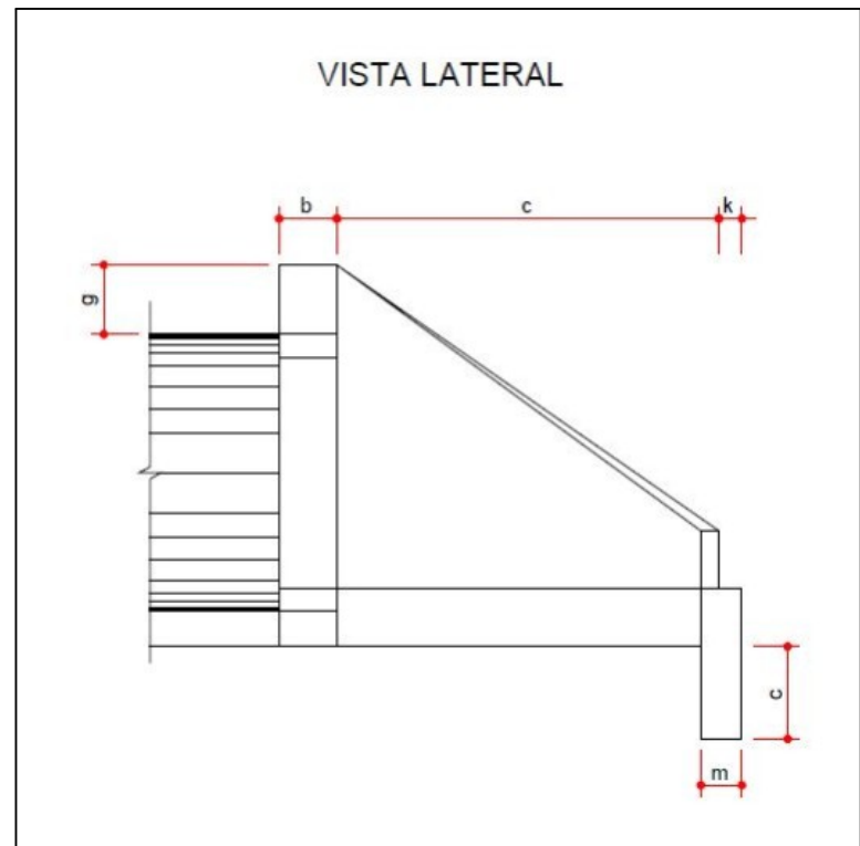
DETALHES - BOCA PARA BUEIRO SEM ESCALA
